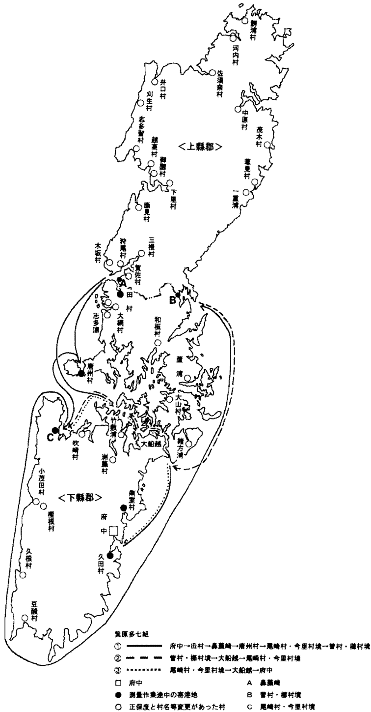
図2 箕原多七組の外廻り海辺測量ルート
