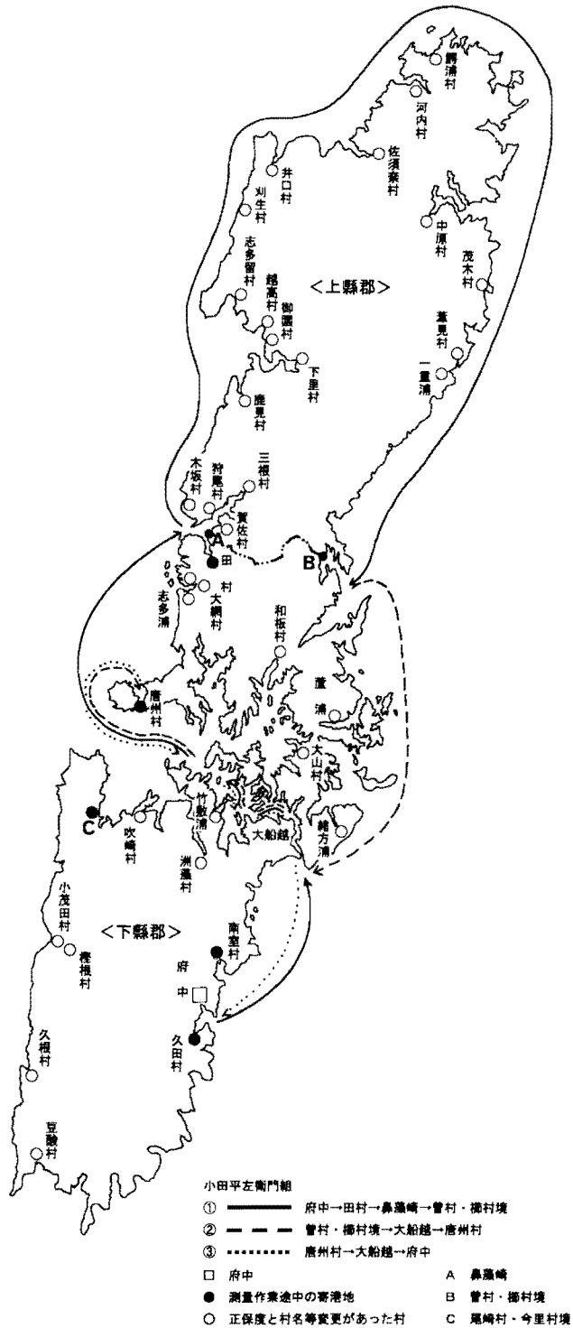
図1 小田平左衛門組の外廻り海辺測量ルート
